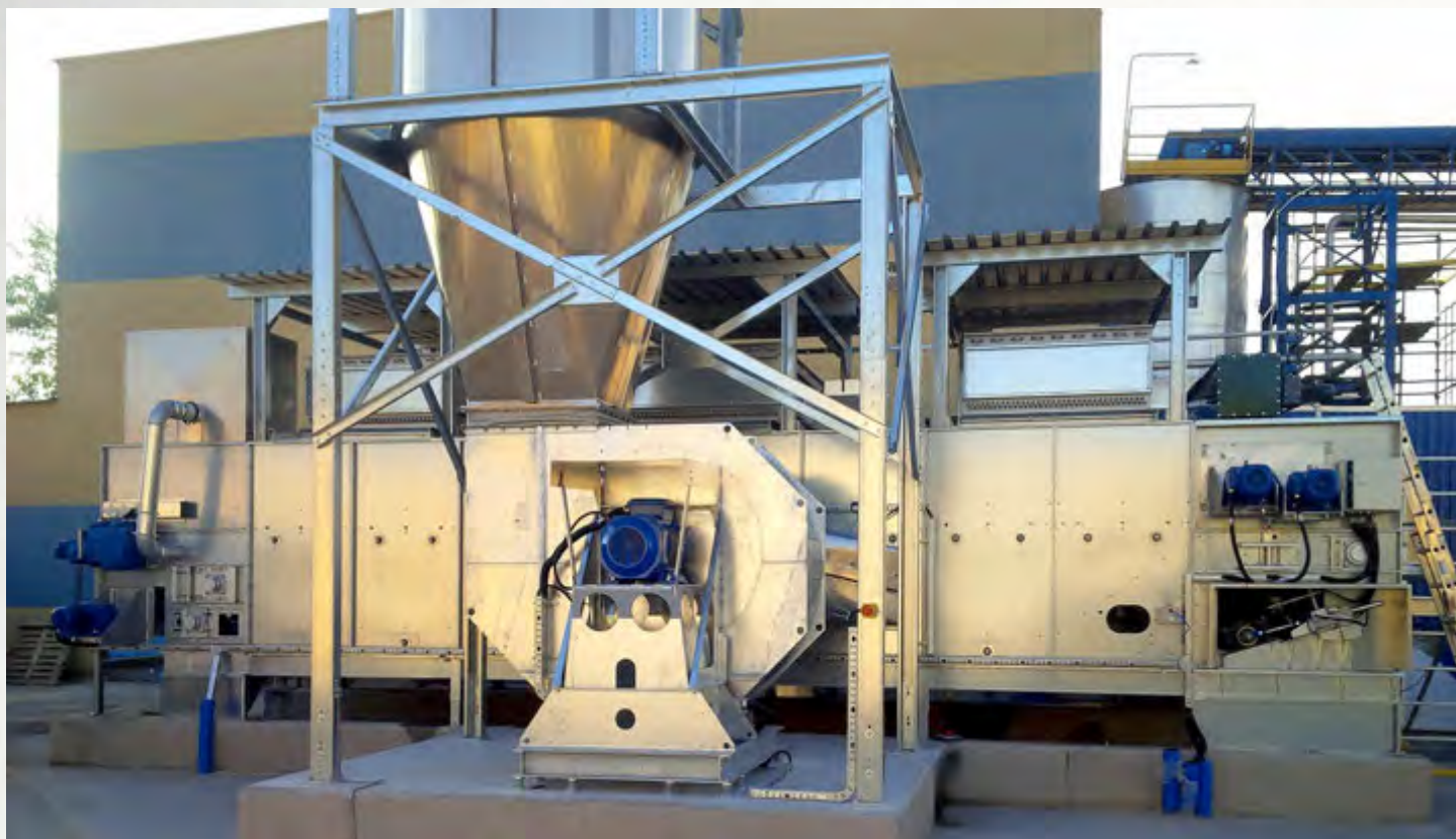
项目地：PPH Tor-Pal Sp.Z.o.o., 波兰 | 型号：BTL 1/3000-8 | 安装年份：2015 干燥物料：木屑 | 出料能力：约1.3吨/小时 | 降水区间：50% - 5%湿度
